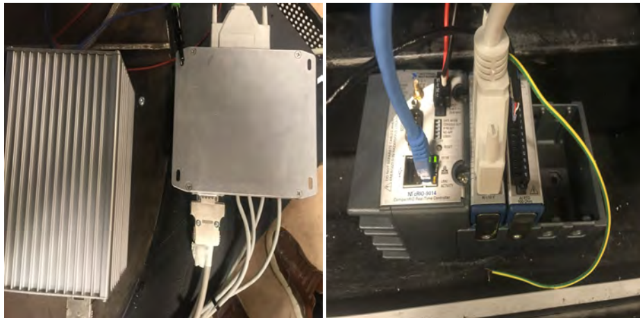
(a) Mätssystem inkopplat i testtrigg.
